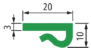
■ GP 261 LK Profile 40M/Roll 型墊片 40M/捲
