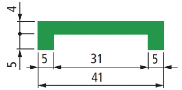
■ GP 362 □ Profile 6M/PCS 型墊片 6M/支
