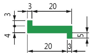
■ GP 262 大Z Profile 45M/Roll 型墊片 45M/捲
